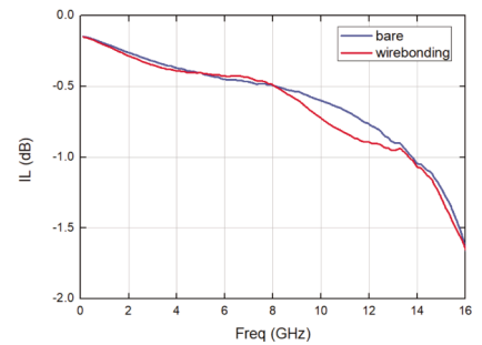
带外抑制 VS 频率
