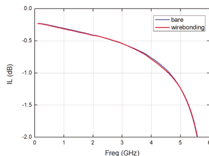
带外抑制 VS 频率
