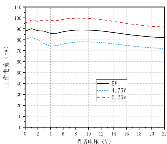
供电电压与工作电流(T=25°C)
