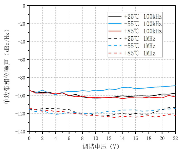
SSB 相位噪声与调谐电压 (Vcc=+5V)
