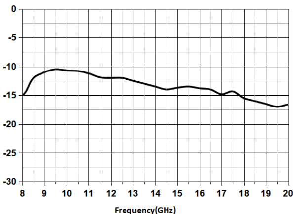
变频损耗 VS 频率
