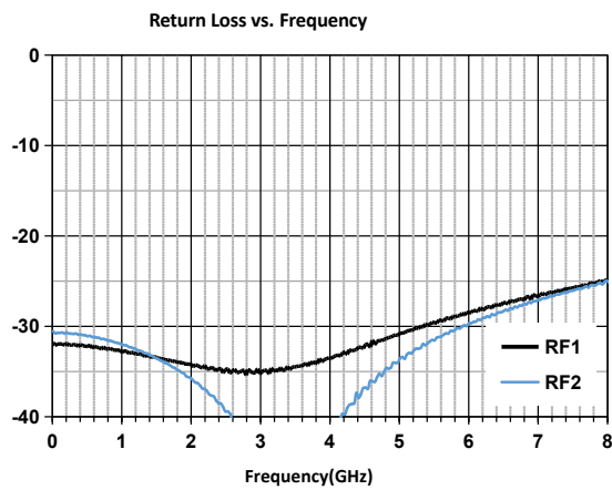
回波损耗 VS. 频率
