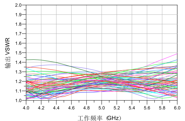
输出驻波 VS 频率
