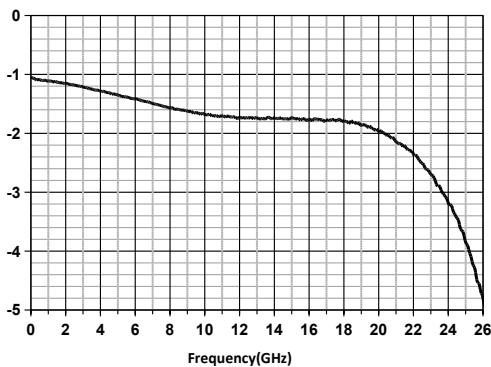
回波损耗(开态) VS 频率
