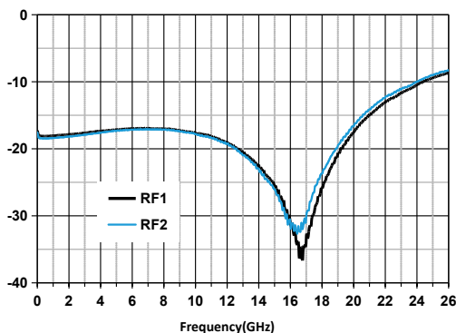
回波损耗(开态) VS 频率
