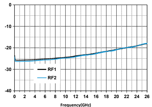
回波损耗(关态) VS 频率
