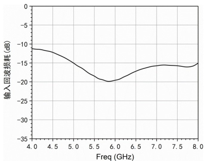
输入回波损耗 VS 频率
