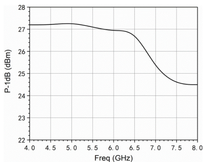
P-1dB VS 频率
