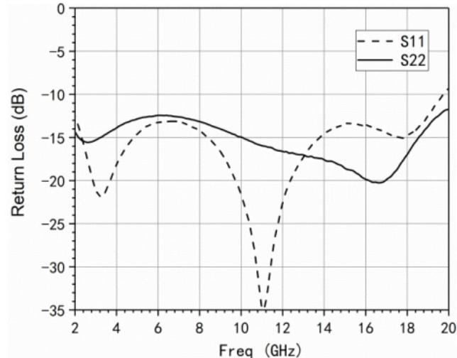
回波损耗 VS 频率
