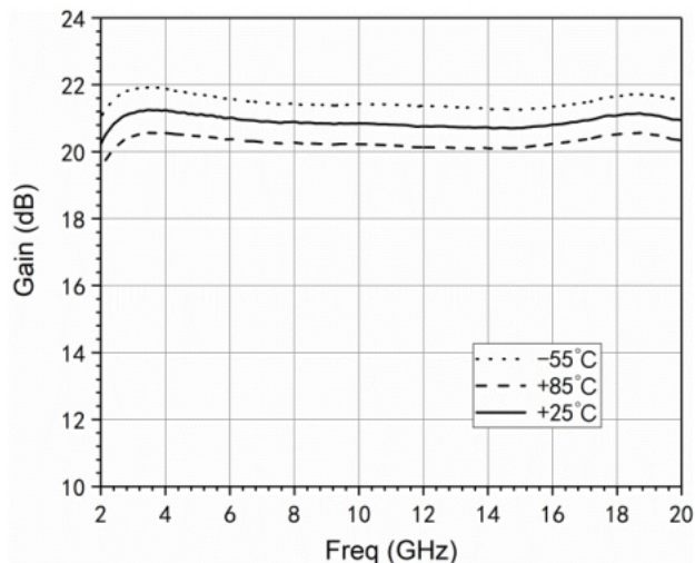
增益 VS 频率
