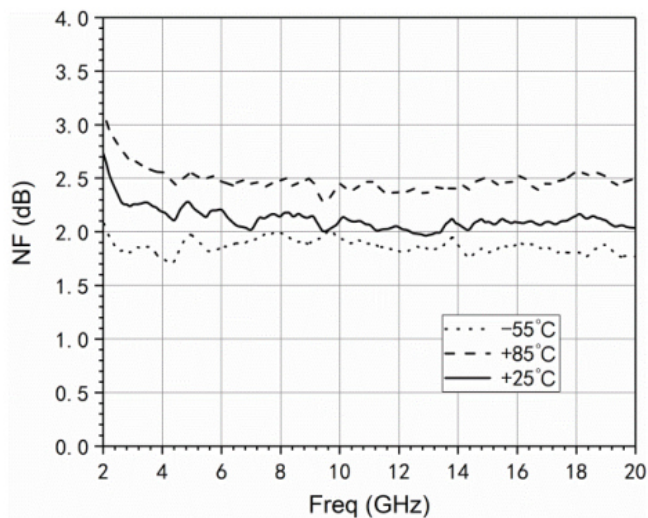
噪声系数 VS 频率
